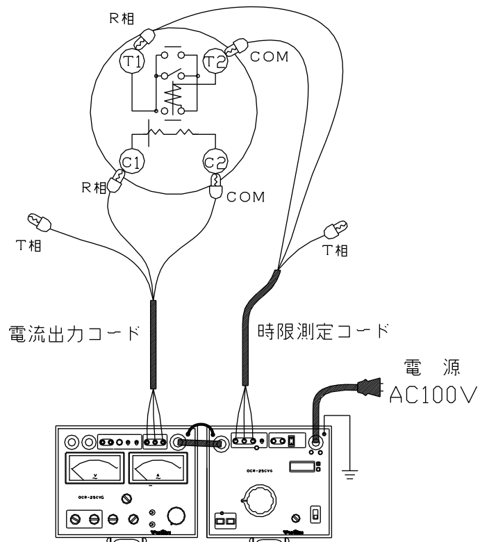
図7：試験回路図－R相単体試験（無電圧引き外し方式）
