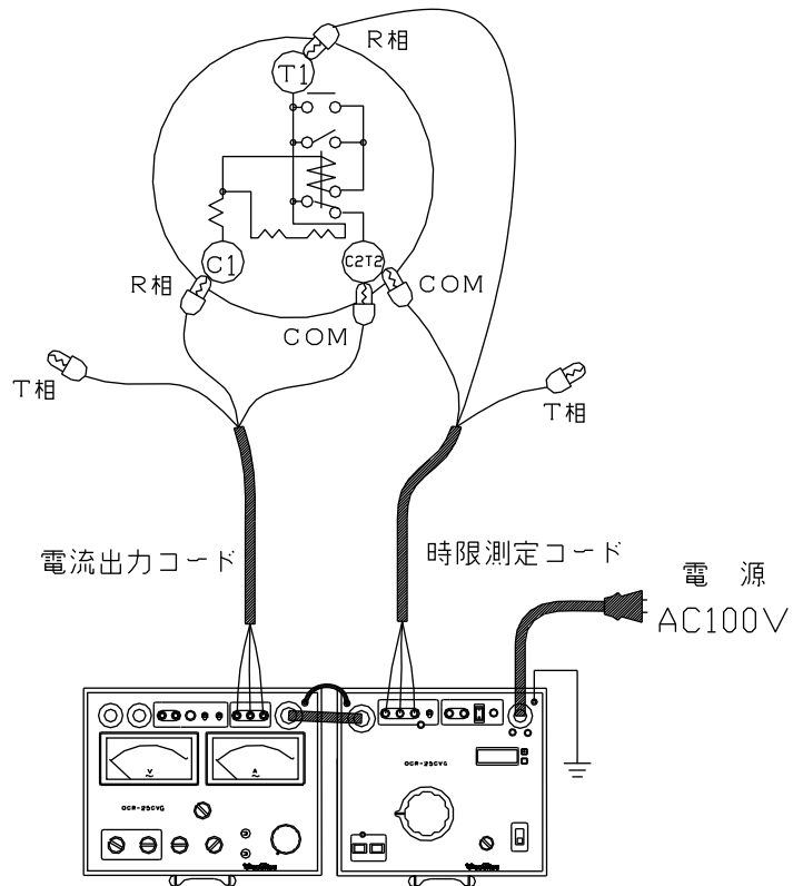
図6：試験回路図－R相単体試験（2次電流引き外し方式）
