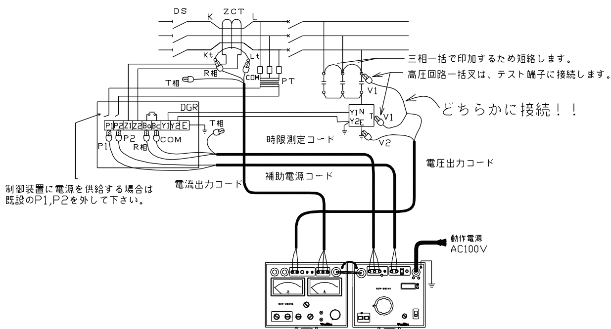
図16：試験回路図－電気室の単体試験（停電状態）
