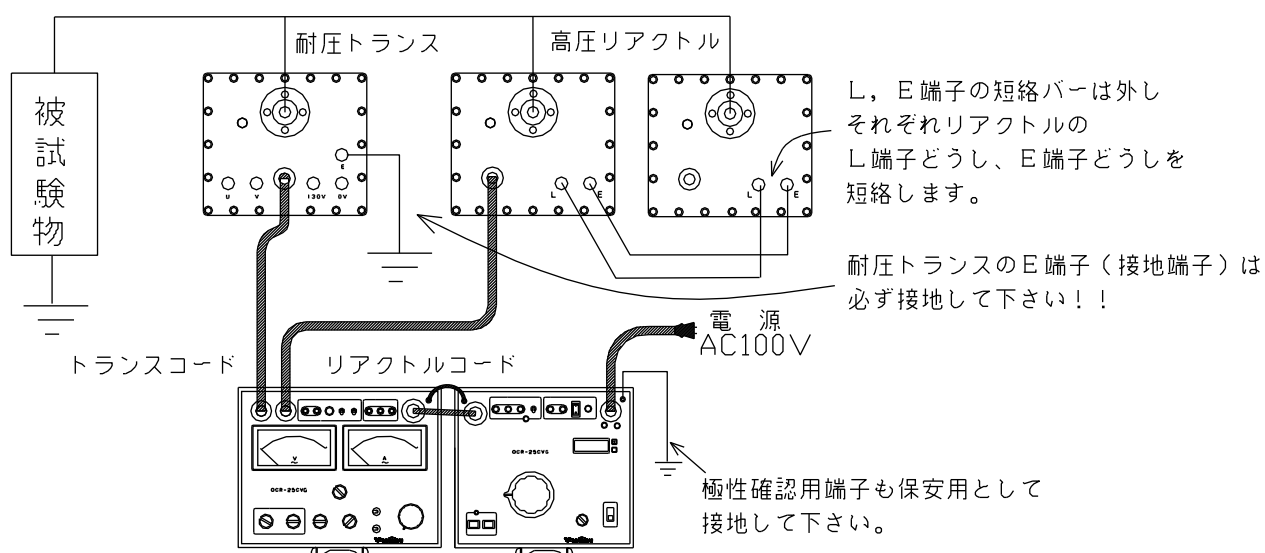
図20：リアクトルを複数使用する場合
