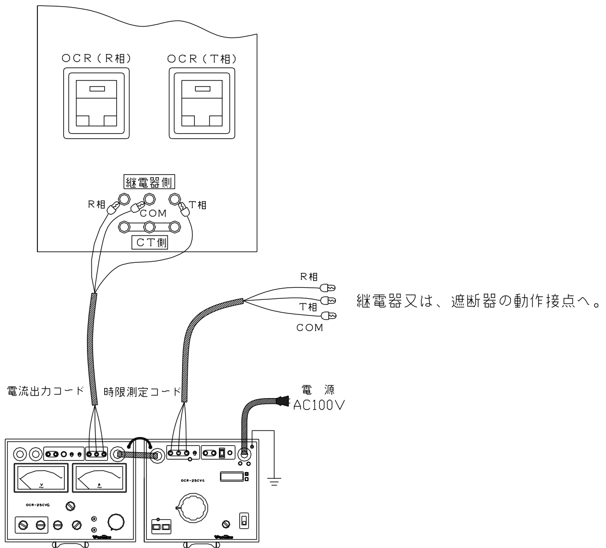
図5：試験回路図（構成）
