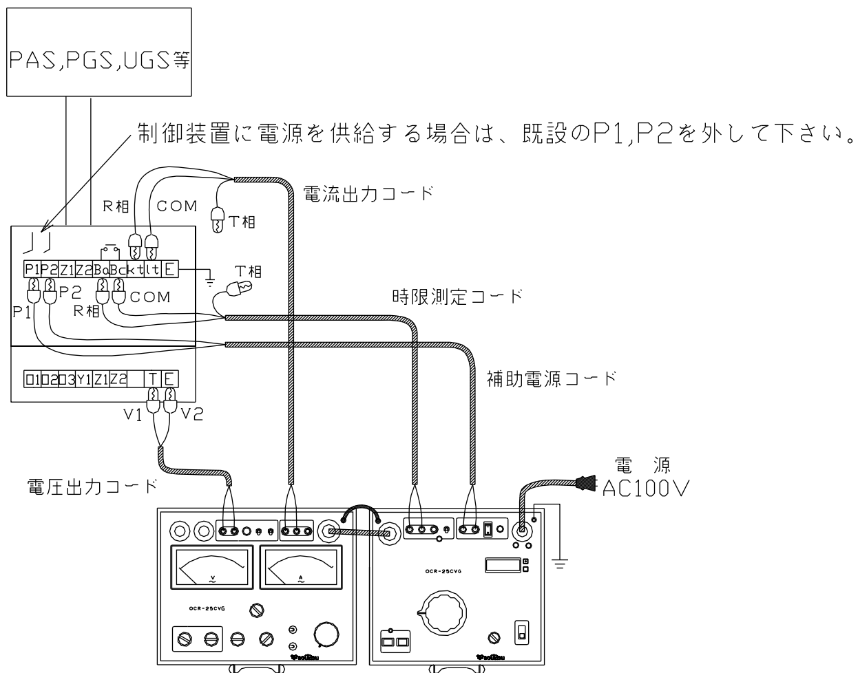
図 1 7：試験回路図－PAS,PGS等の単体試験（停電状態）
