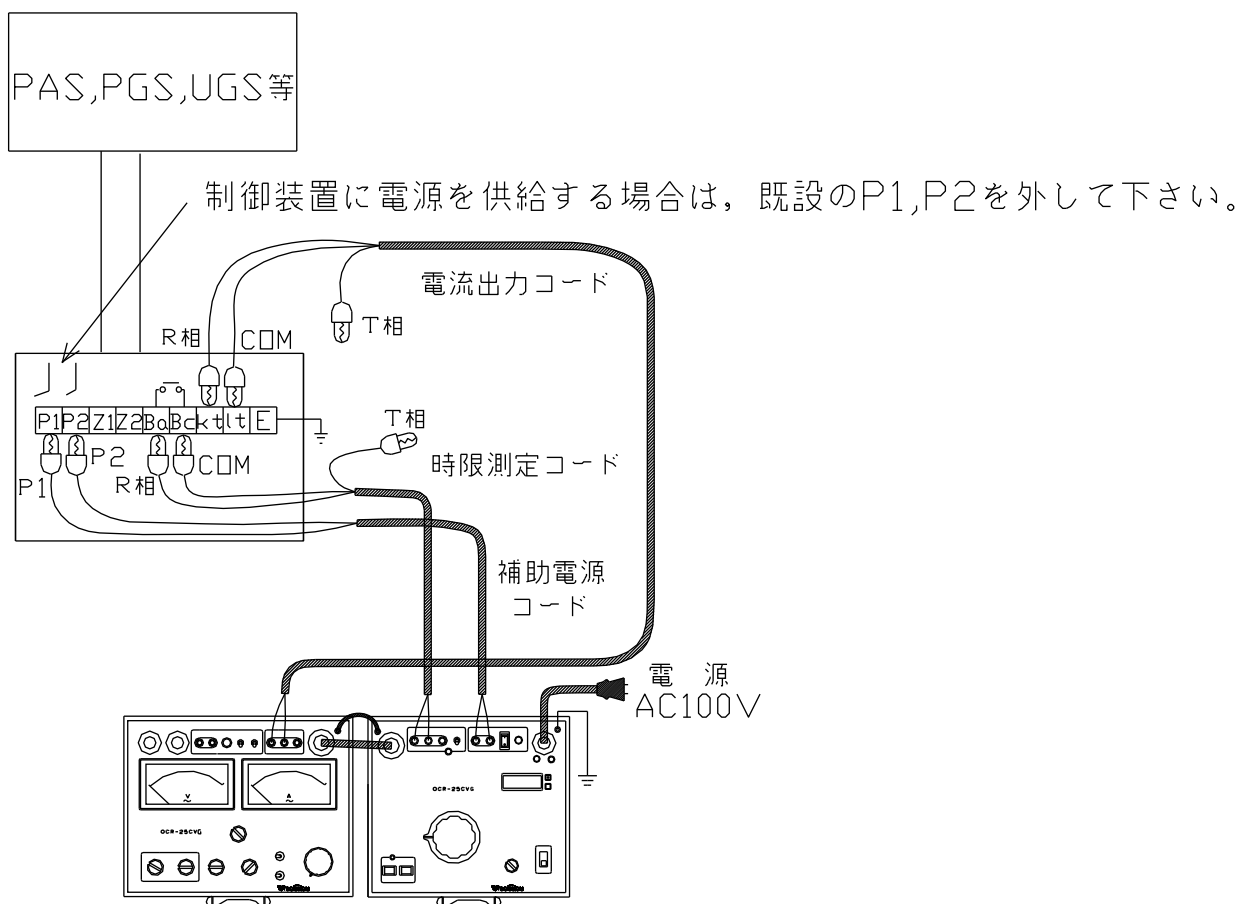
図15：試験回路図－PAS,PGS等の単体試験（停電状態）
