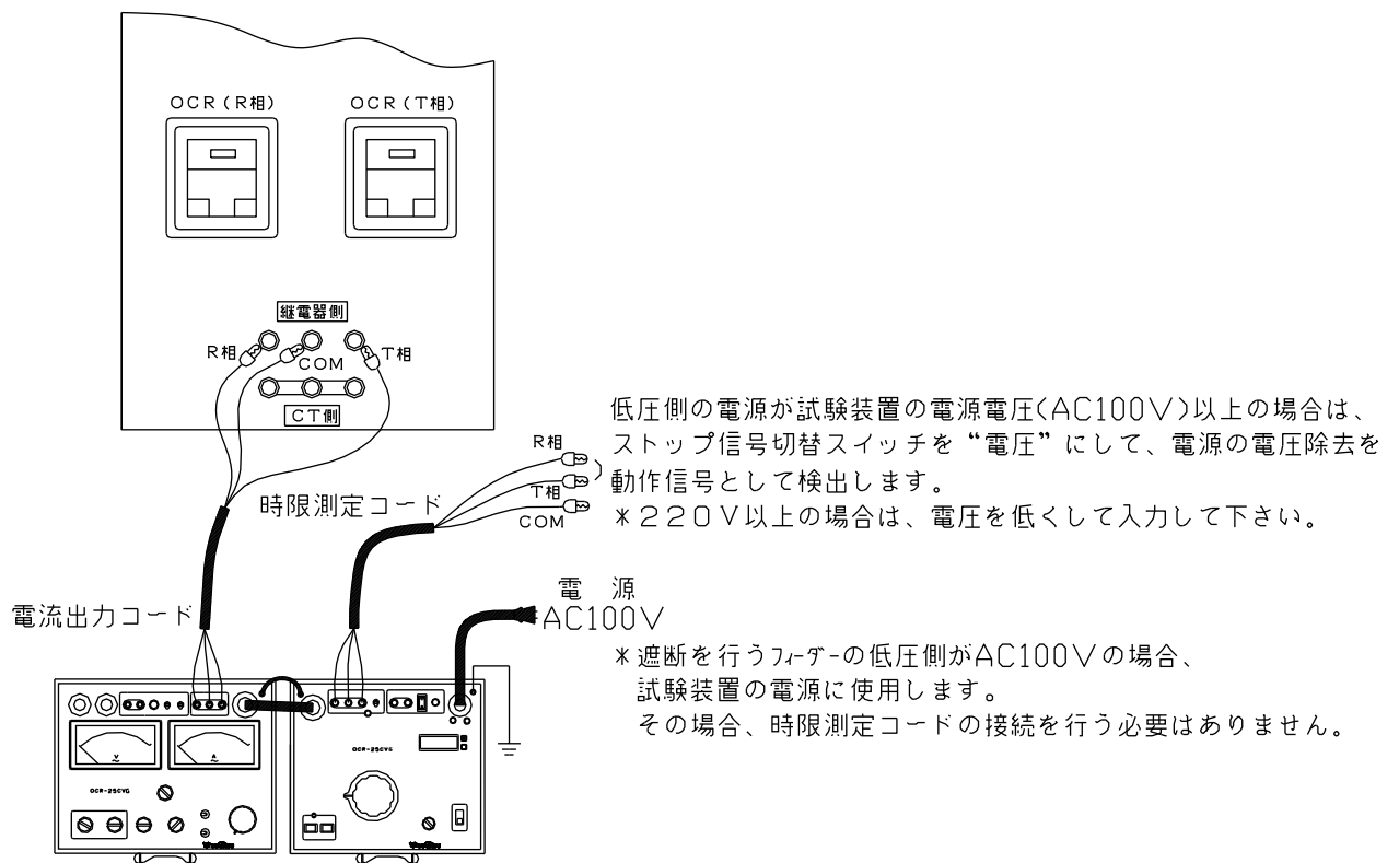
図9：試験回路図一連動試験（受電状態）
