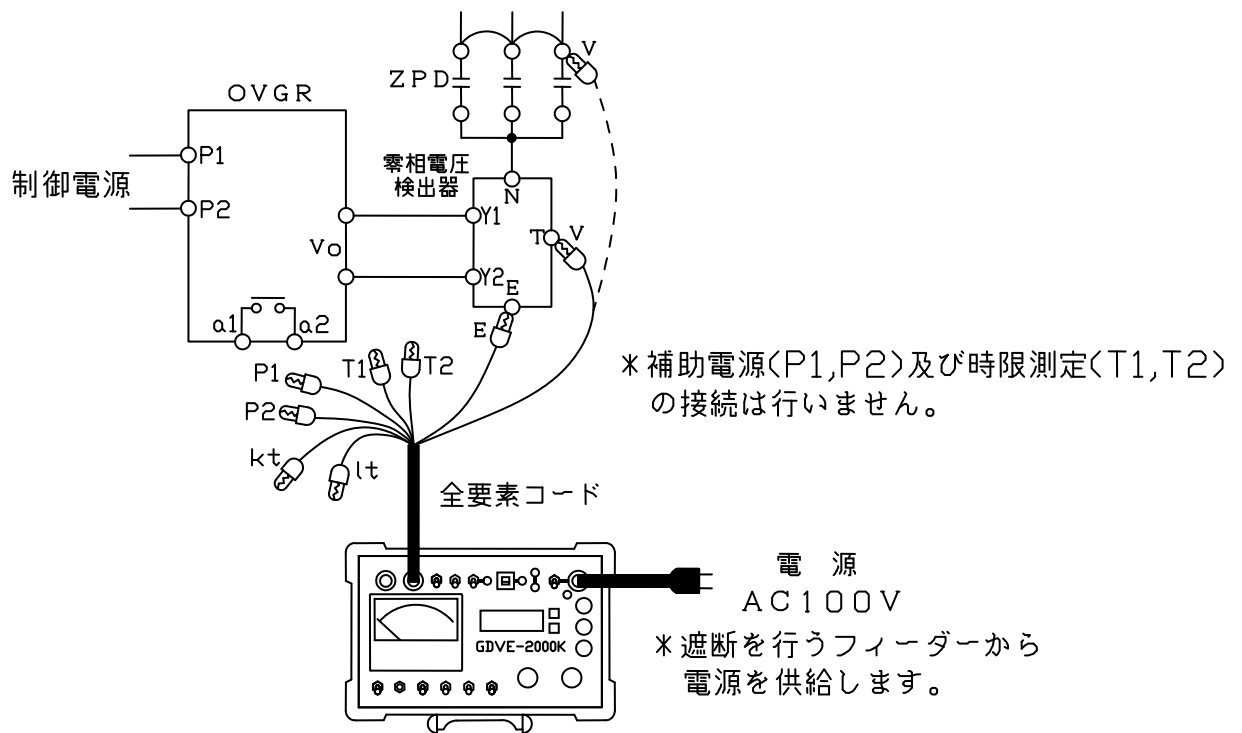
図8：試験回路図一連動試験（受電状態）
