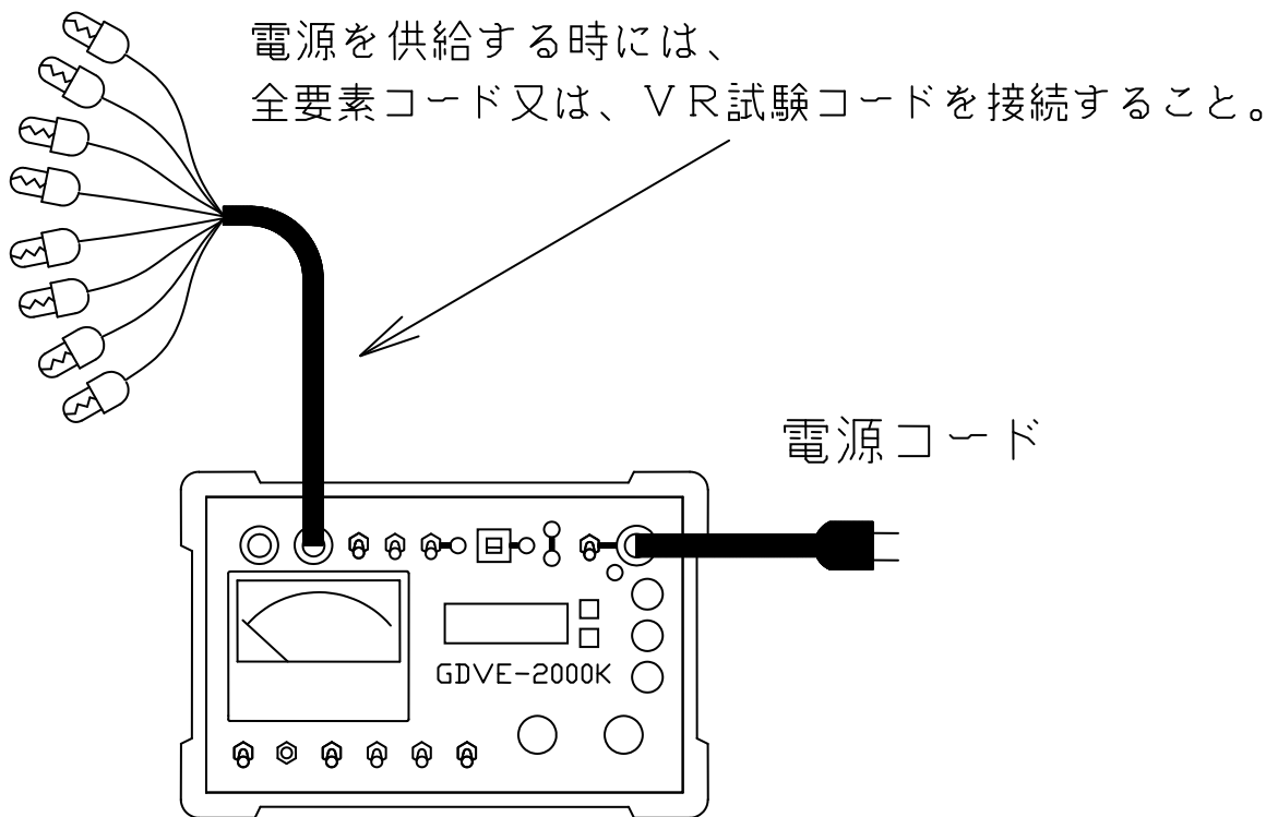
図1：電源の供給
