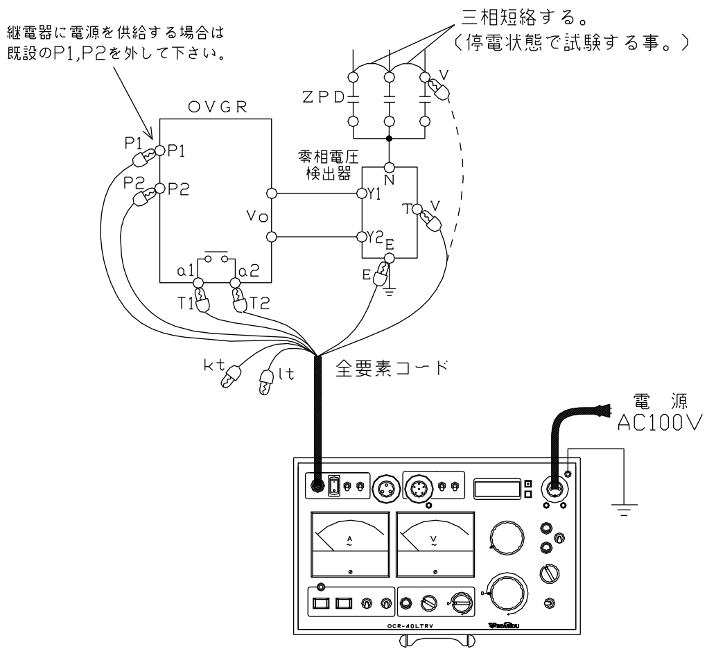
図17: OVGRの試験回路図
