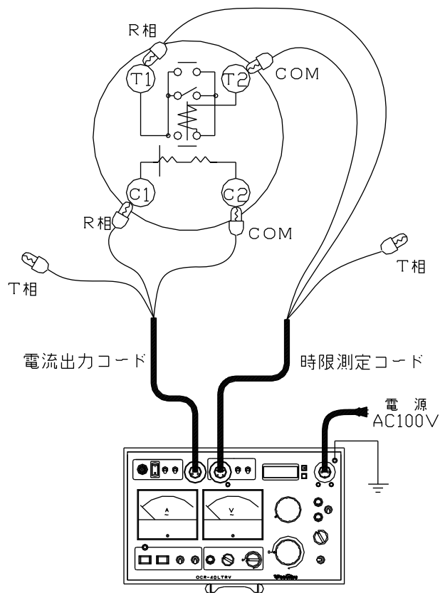
図8：単体試験（無電圧引き外しタイプ：R相）
