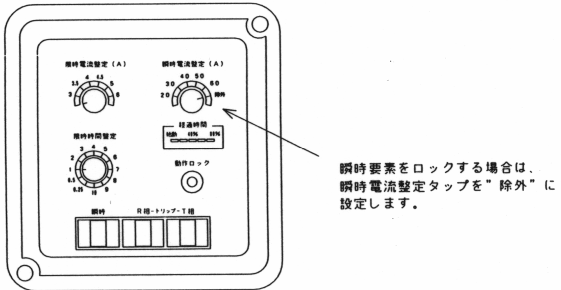
図11：瞬時要素のロック方法（静止形）
