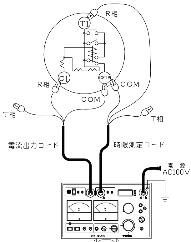
図6：単体試験（2次電流引き外しタイプ：R相）時限測定コード接続有り
