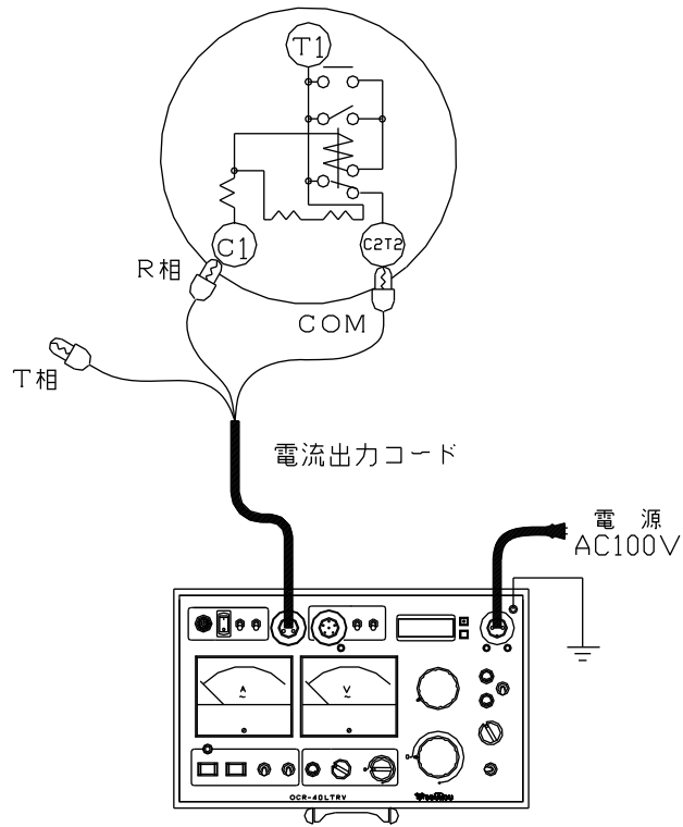
図7：単体試験（2次電流引き外しタイプ：R相）時限測定コード接続無し
