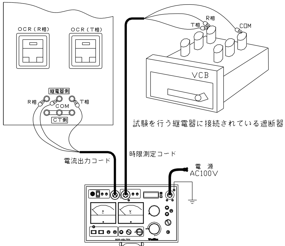
図9：連動試験（停電状態）
