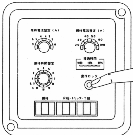
図13：限時要素のロック方法（静止形）
