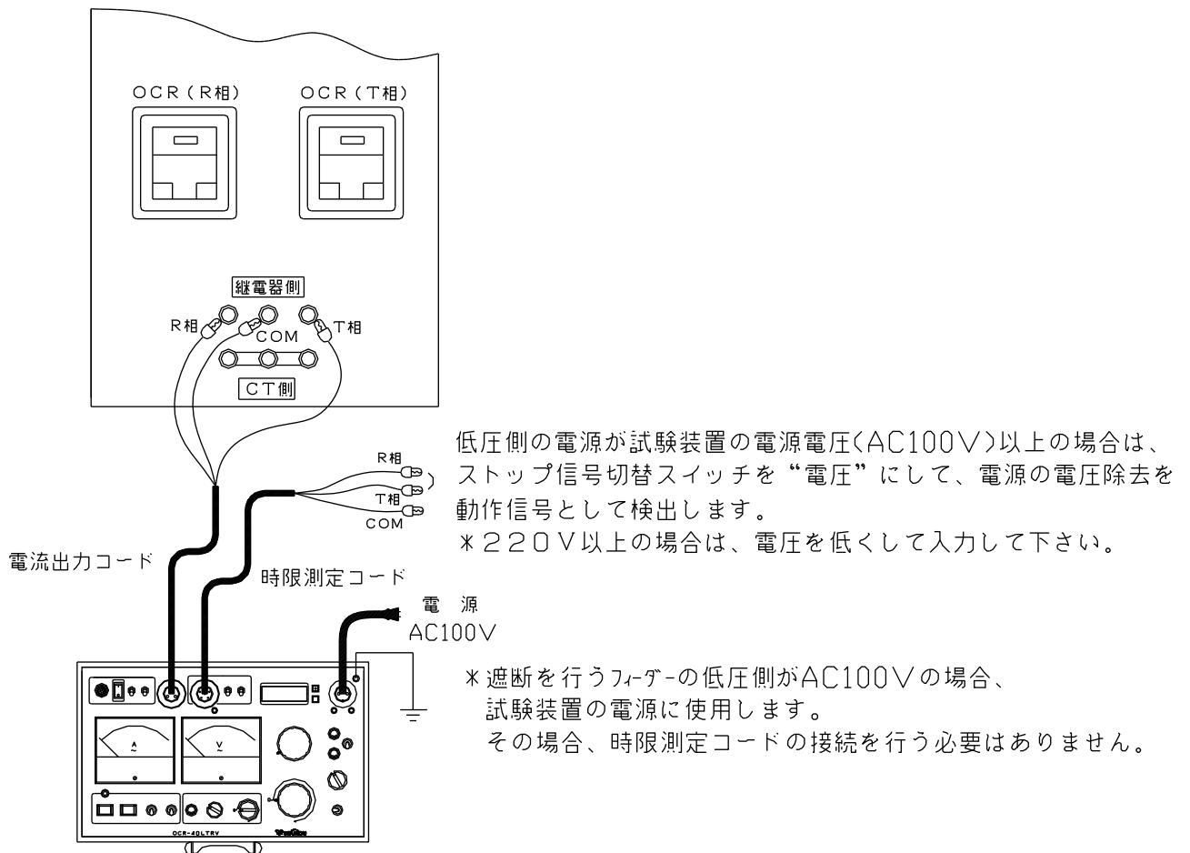
図10：連動試験（受電状態）
