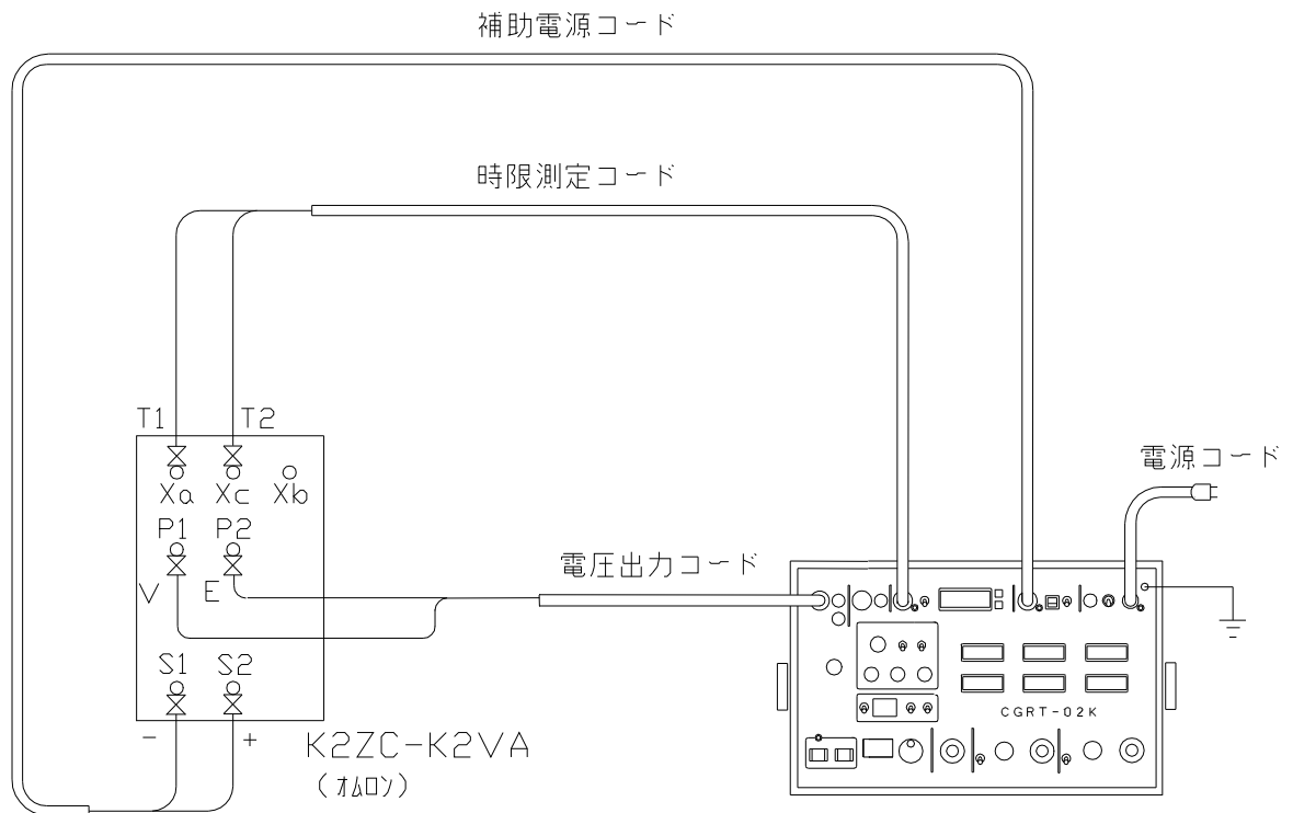
図4：過電圧継電器の接続
