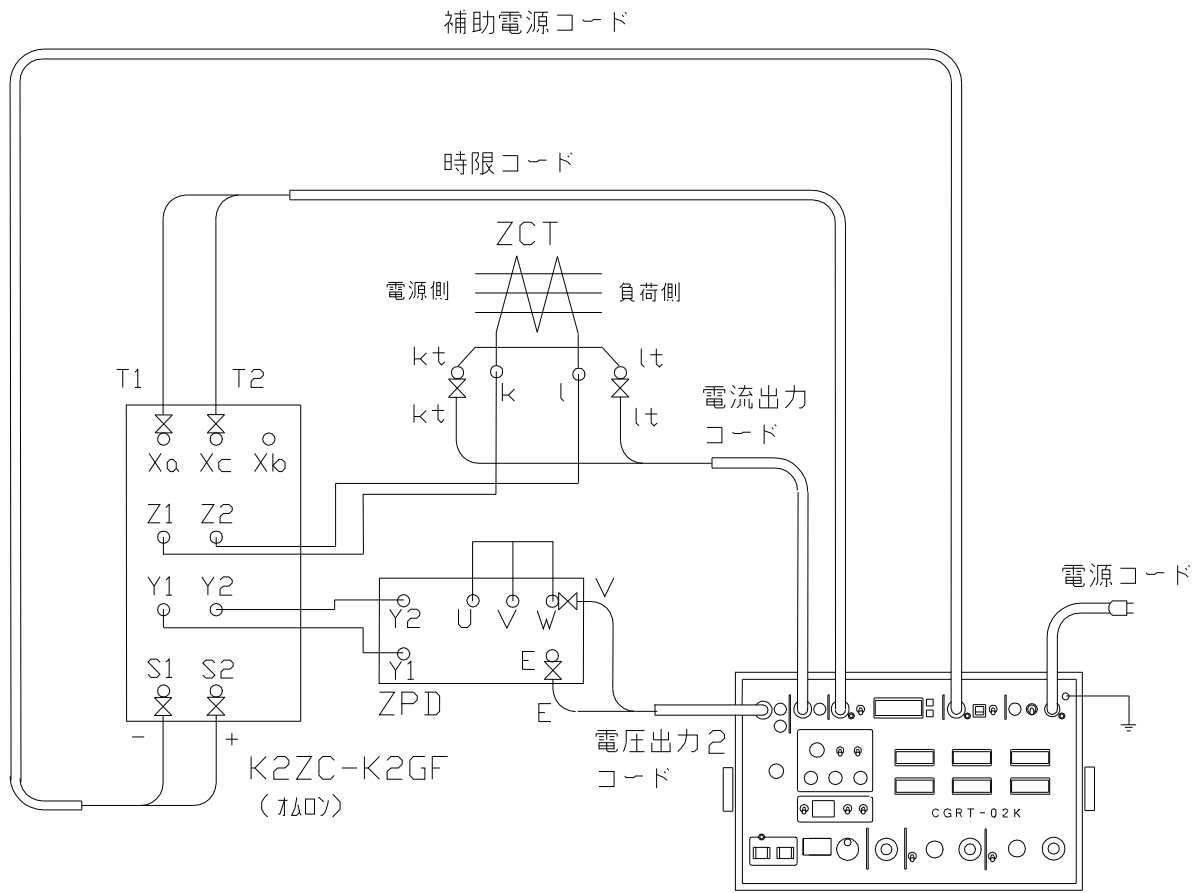
図1：方向性地絡継電器の接続
