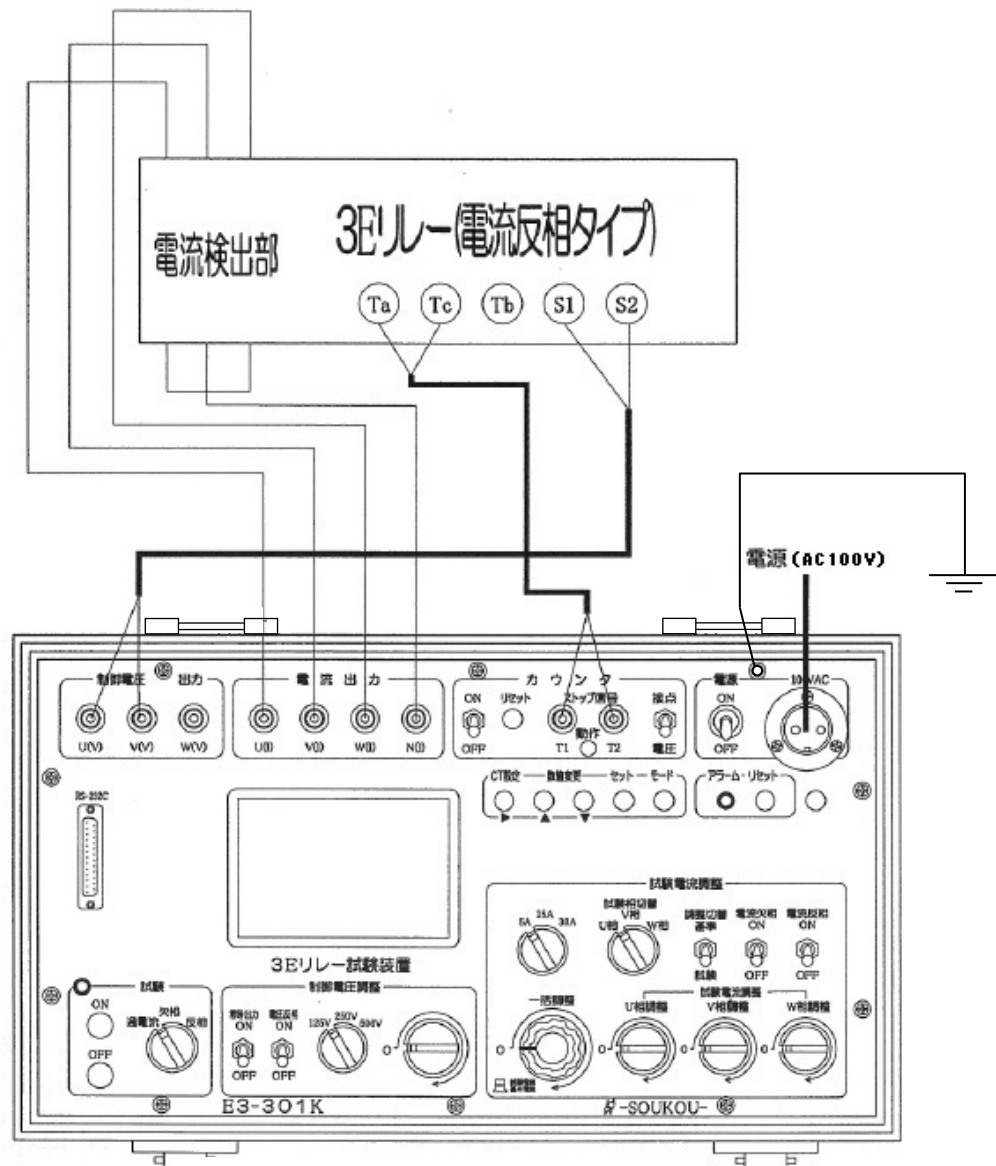
図1：試験回路図（電流反相タイプ）
