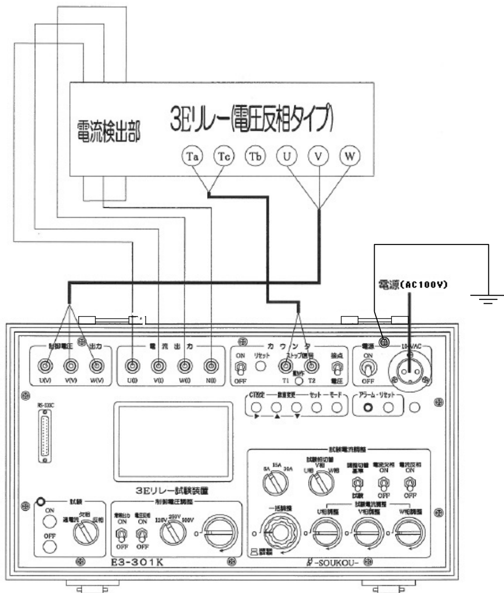
図2：試験回路図（電圧反相タイプ）
