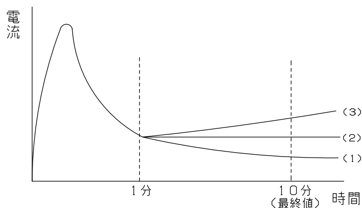
図6：電流の時間的变化（成極比）
