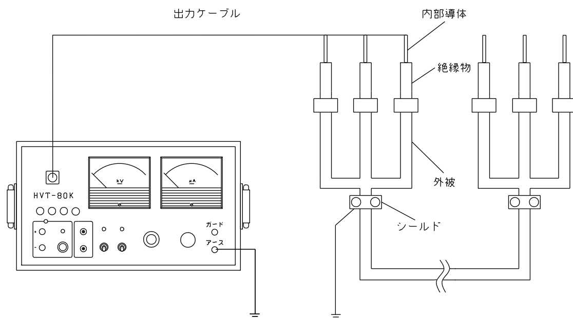
図1：ケーブルの絶縁耐力試験接続方法
