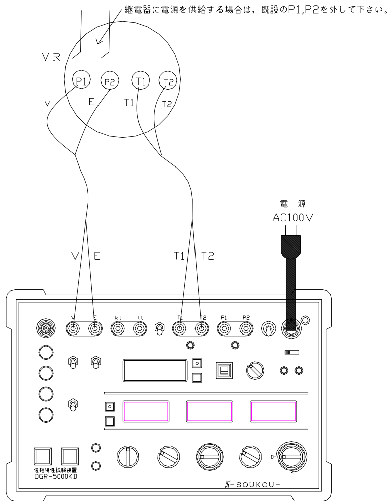
図9：OVR,UVRの試験回路図
