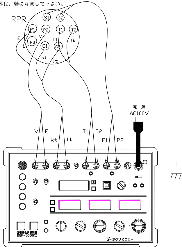
図 10 : RPRの試験回路図
