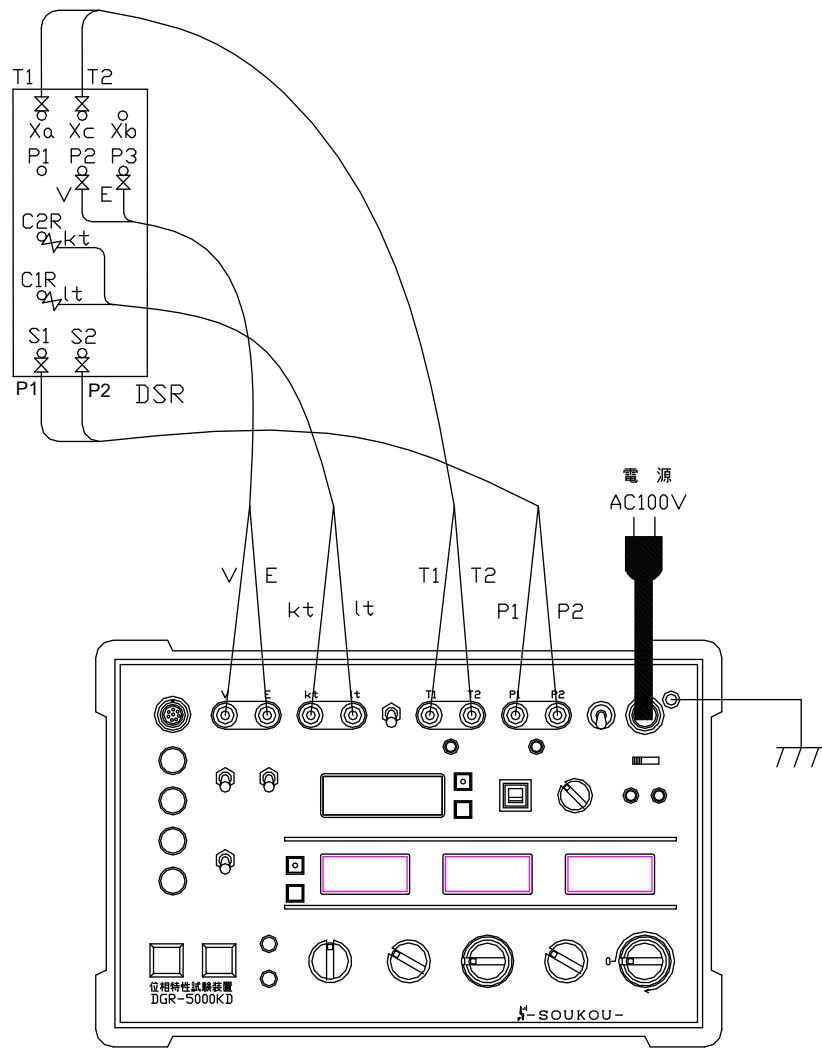
図 10 : DSRの試験回路図(K2ZCの例)
