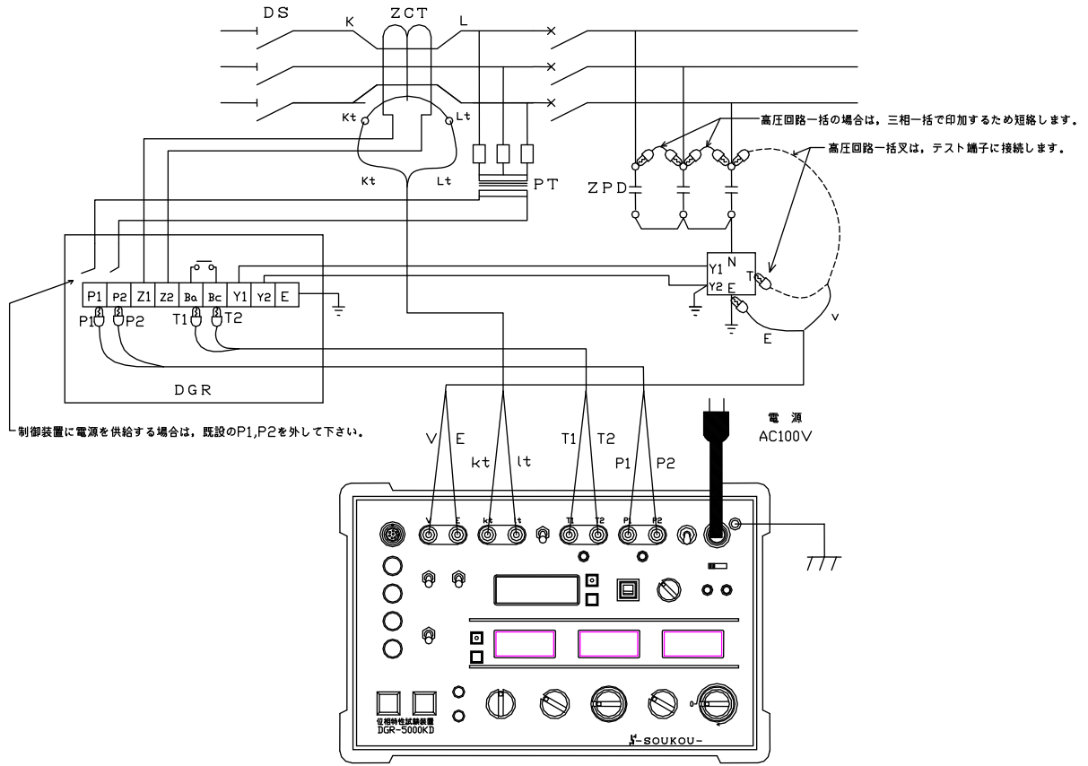
図3：試験回路図—電気室等のDGRの単体試験（停電状態）
