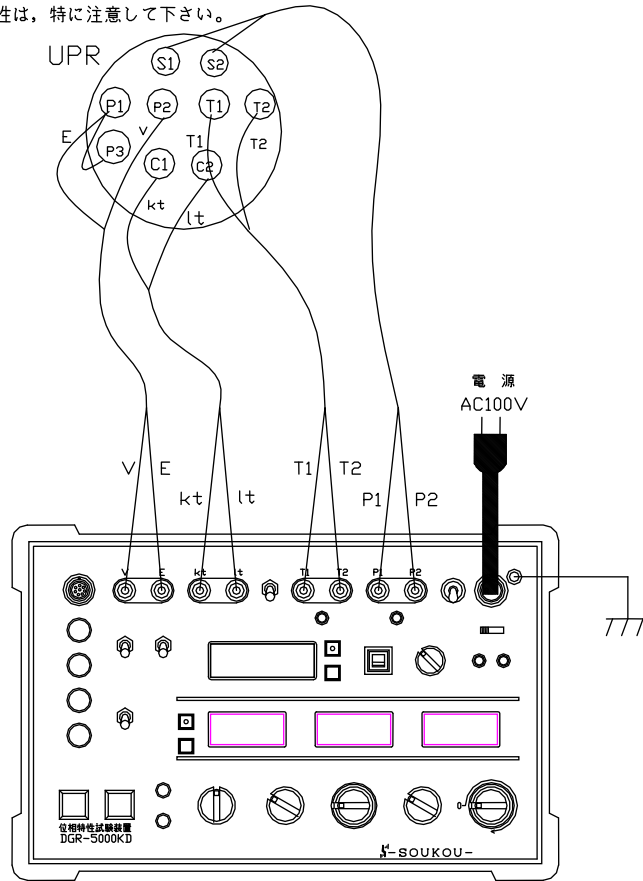
図 11 : UPRの試験回路図
