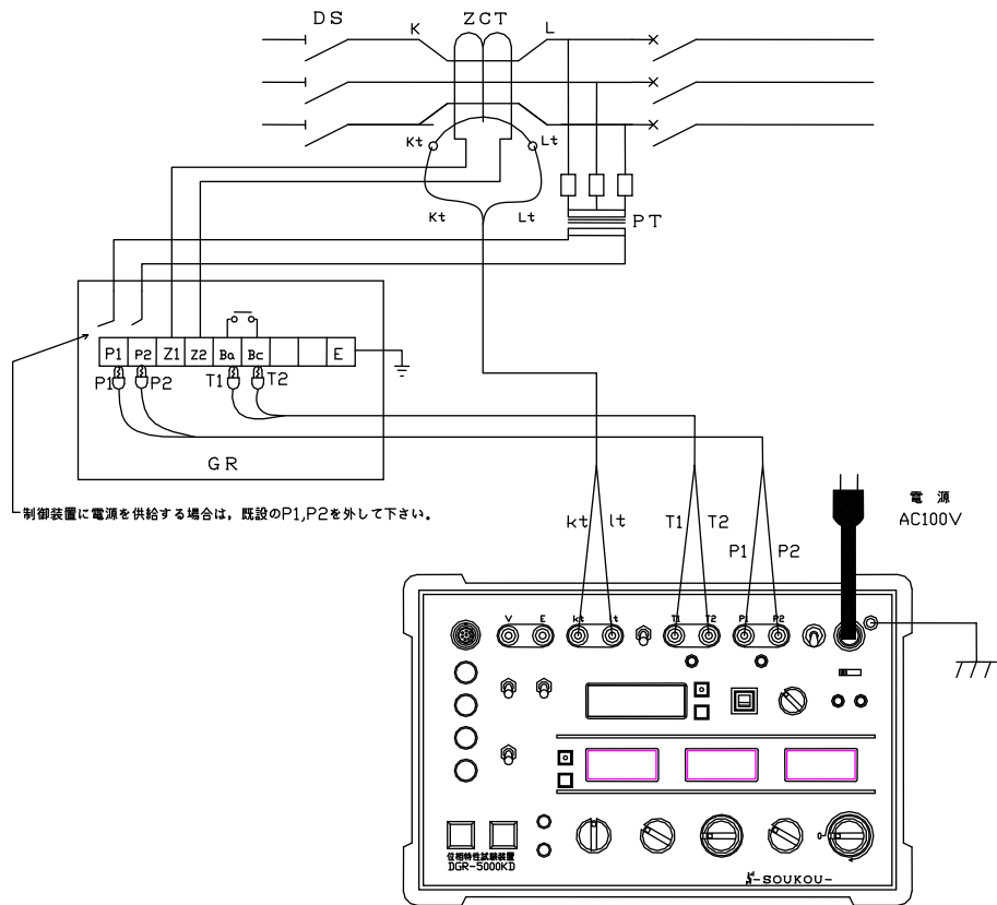
図6：試験回路図一電気室等のGRの単体試験（停電状態）
