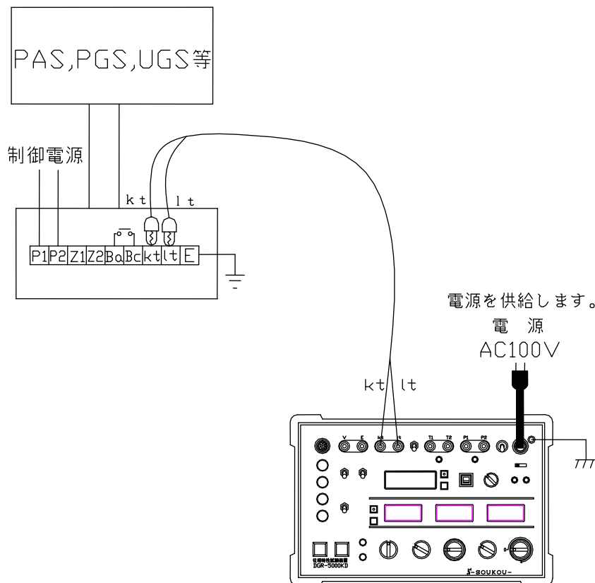
図5：試験回路図—PAS, PGS等の連動試験（受電状態）
