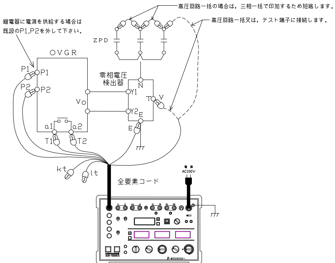
図7：OVGRの試験回路図
