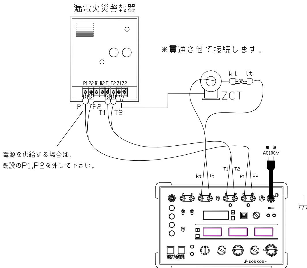
図8：漏電火災警報器の試験回路図
