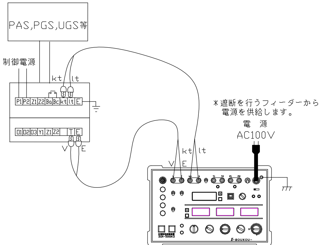
図2：試験回路図—PAS,PGS等の連動試験（受電状態）
