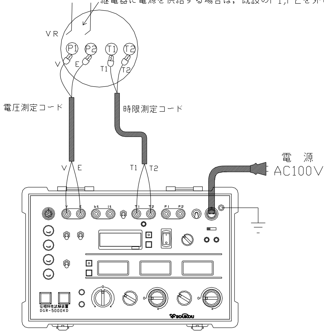
図9：OVR,UVRの試験回路図
