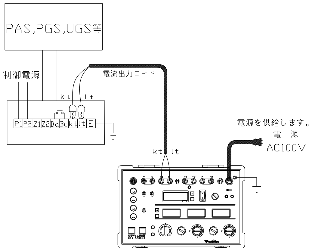
図5：試験回路図－PAS, PGS等の連動試験（受電状態）
