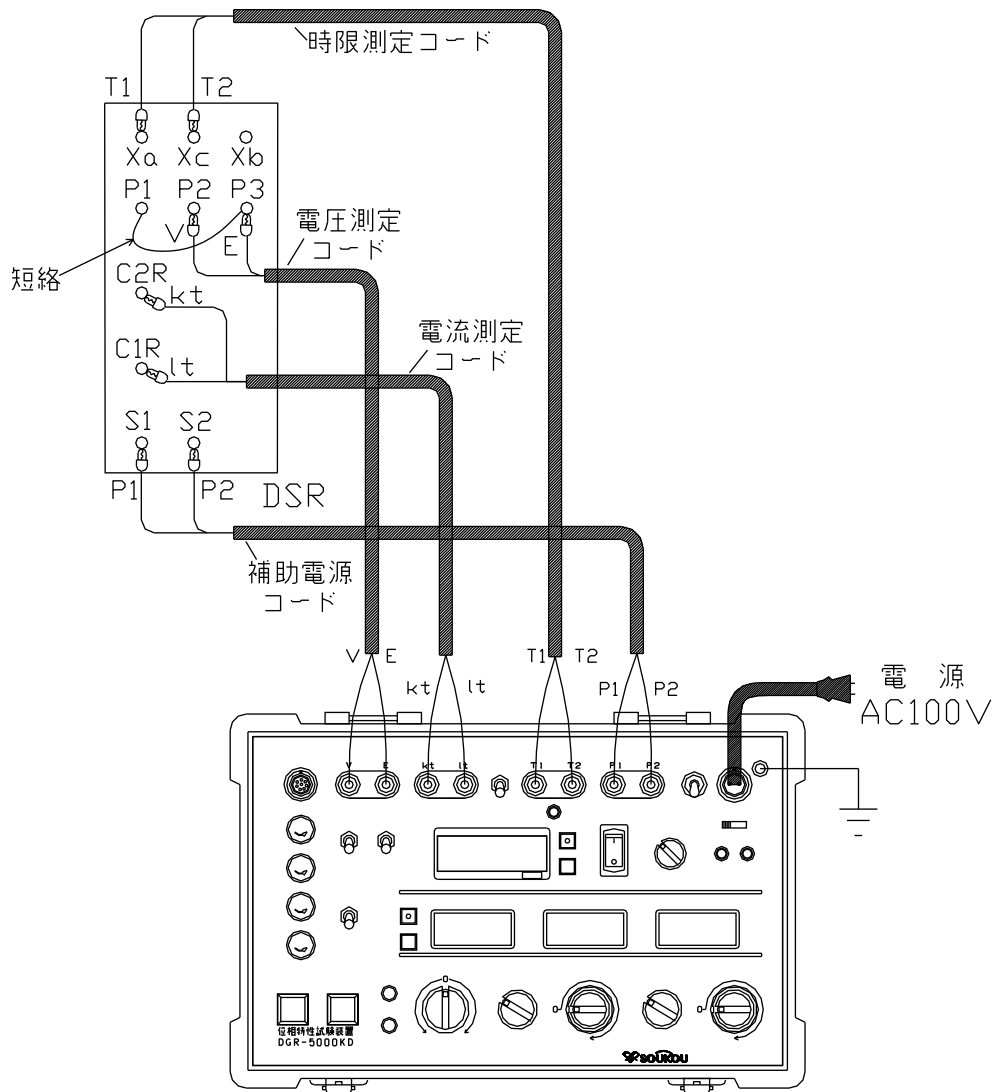
図 10 : DSRの試験回路図 (K2ZCの例,R相試験の接続例)
