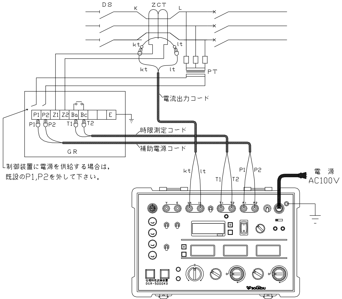
図6：試験回路図一電気室等のGRの単体試験（停電状態）
