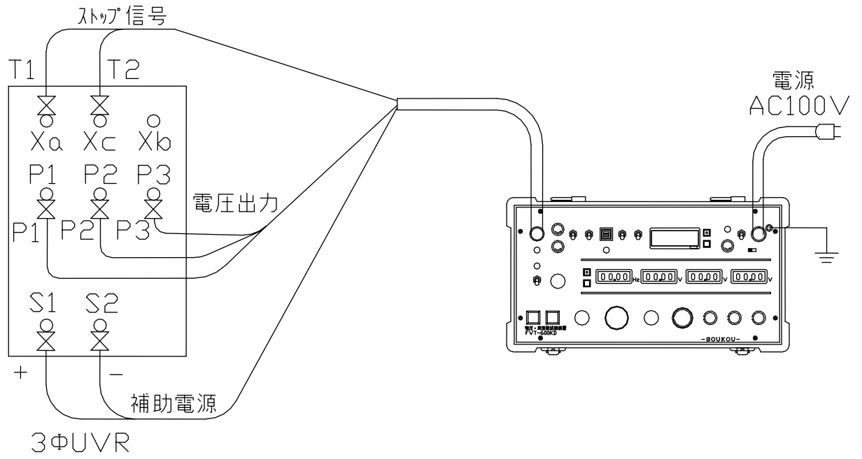
図2：3相UVRの試験回路図
