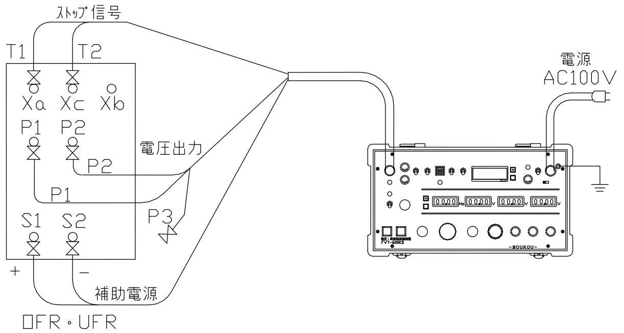
図4：OFR,UFRの試験回路図
