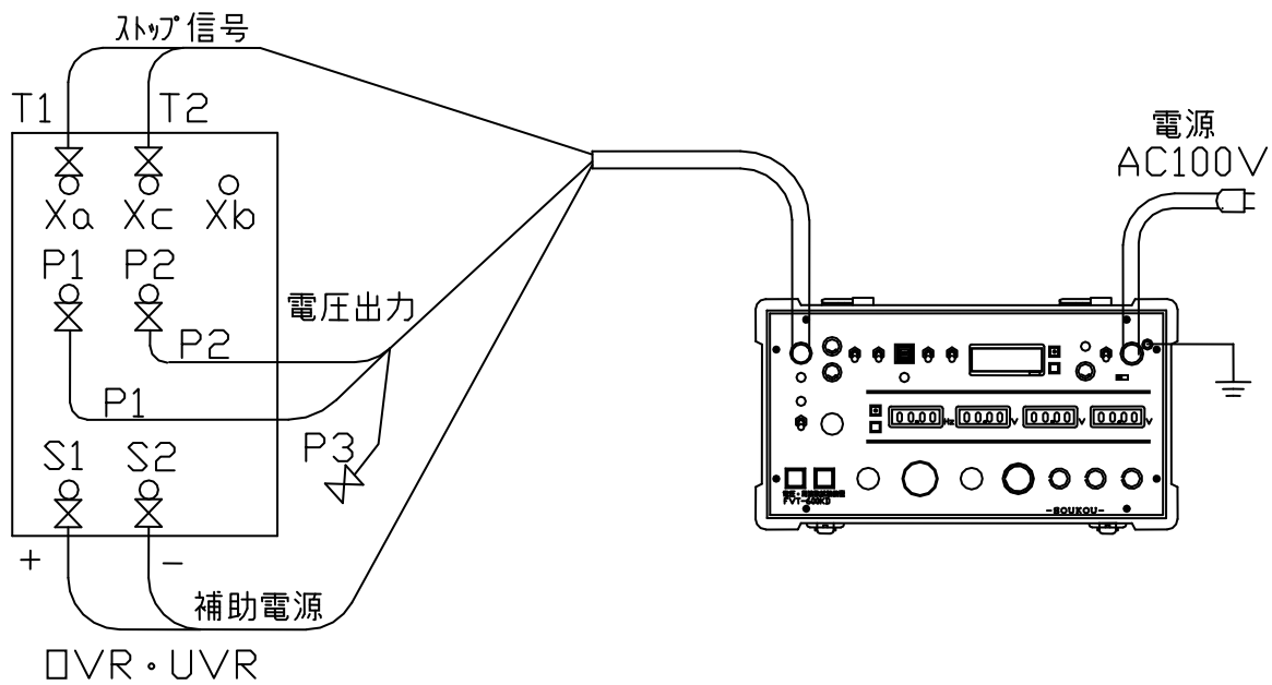
図1：OVR,UVRの試験回路図
