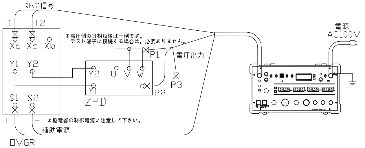
図3：OVGRの試験回路図
